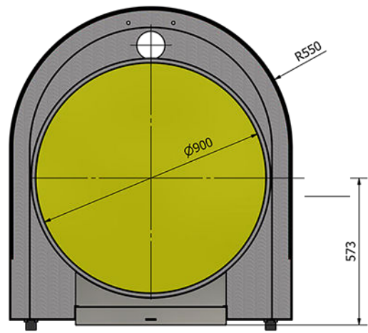
A-A (0,1 : 1)
